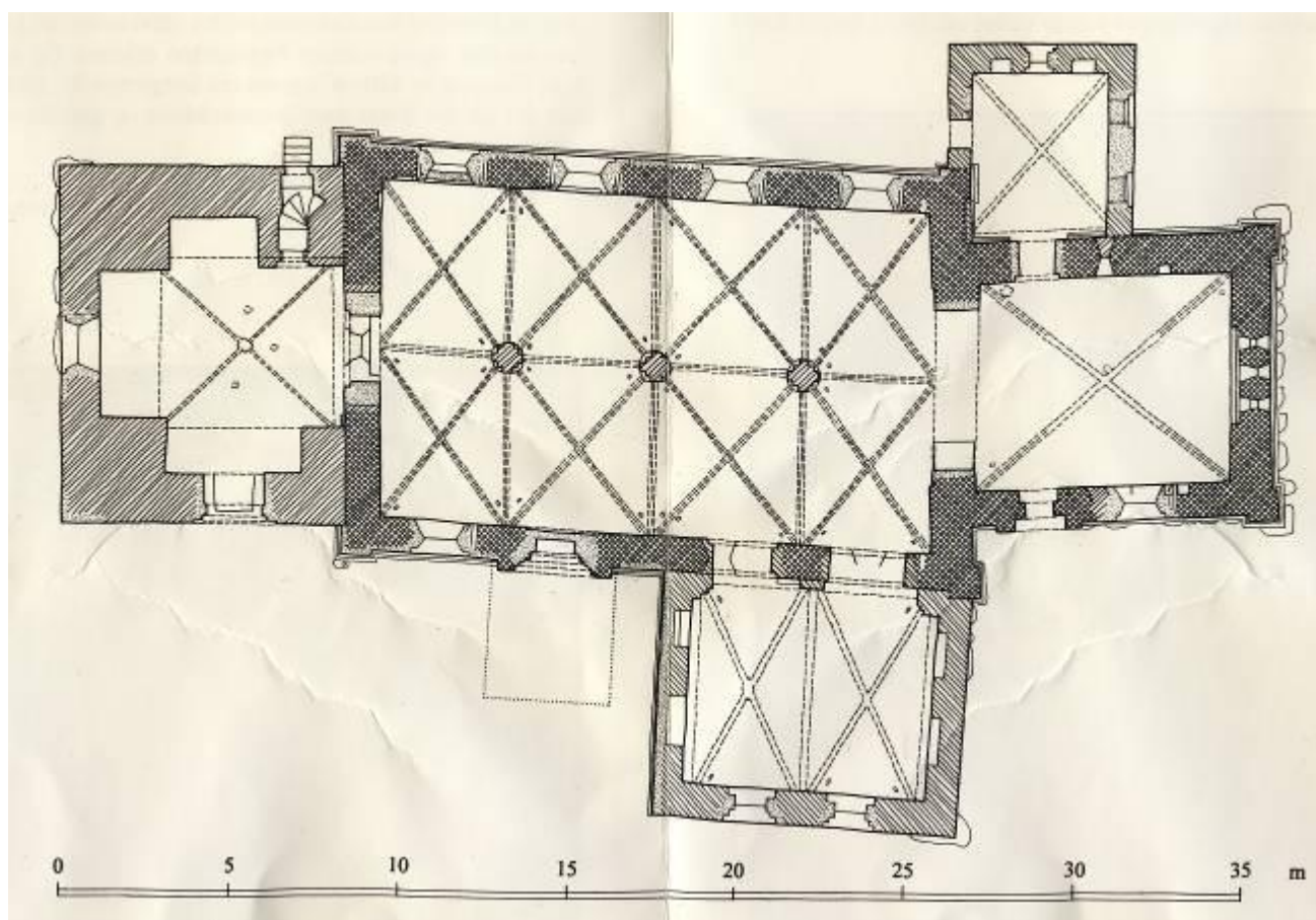
Kirkens grundplan, 1:300.
